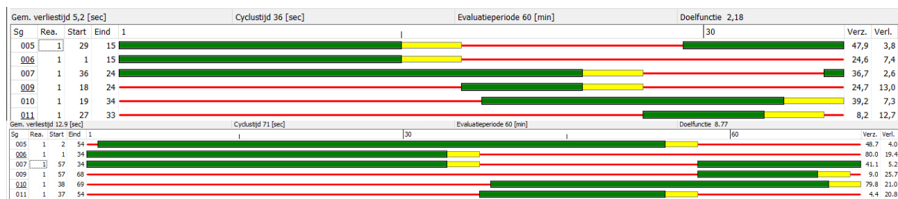
Figuur 10: resultaat COCON berekeningen oostelijk kruispunt aansluiting Heiloo voor de ochtend- en avondspits
